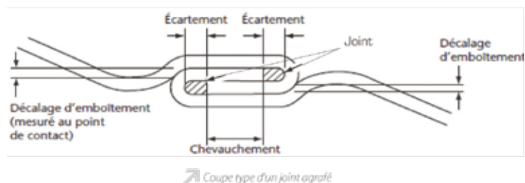
Tuyaux en tôle ondulée à joint hélicoïdal agrafé
