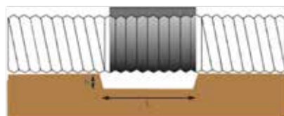
SCHEMA D'UN DÉCAISSEMENT SOUS COLLIER
