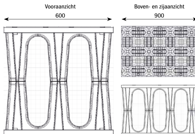
IT PLUS® COLUMNBOX ZONDER GEINSTALLEERD ZIJPANEEL.
