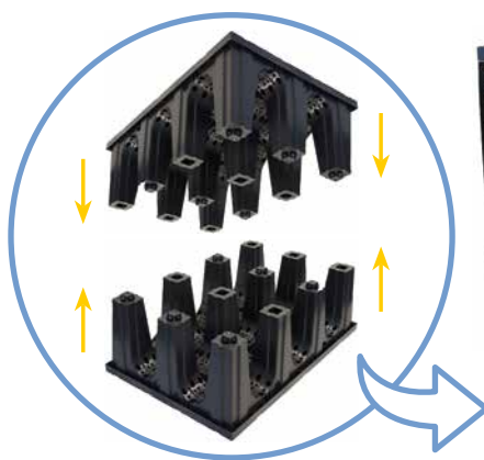
SAMENGESTELDE COLUMNBOX 900 x 600 x 600 mm Art. nr. 32991
